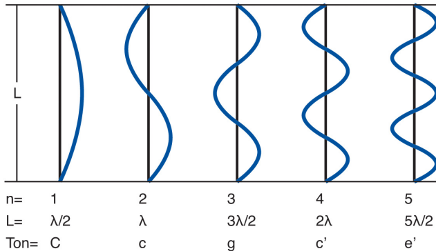
Abbildung 4.3: Oberwellen sind ganzzahlige Vielfache (n) einer Grundfrequenz.
