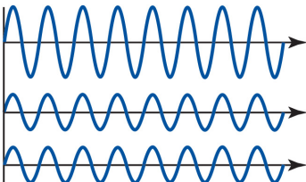
Konstruktive Interferenz
