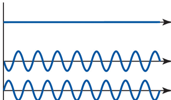
Destruktive Interferenz
