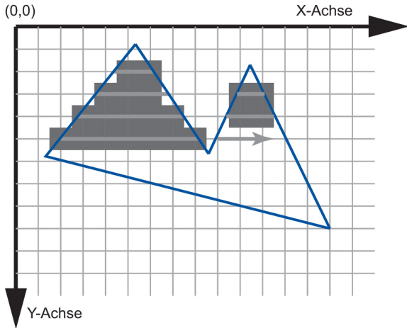
Abbildung 7.12: Ausfüllen eines Polygons mit dem Scanline-Algorithmus
