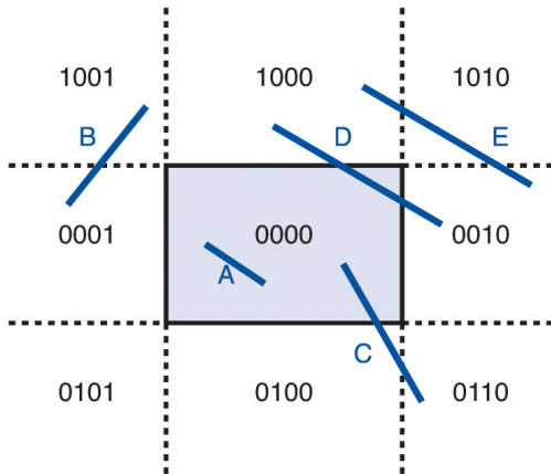
Abbildung 7.7: Line Clipping nach Cohen und Sutherland
