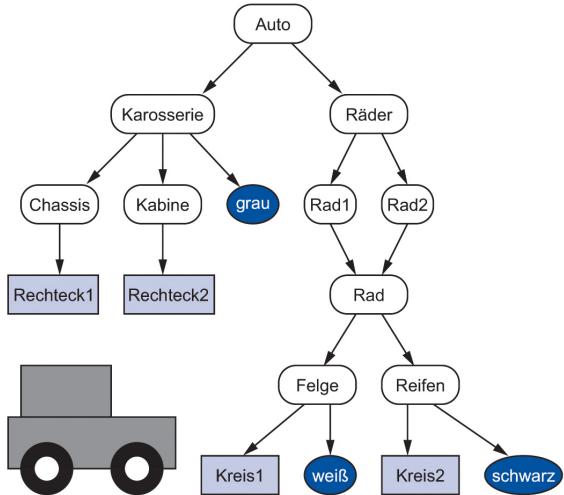
Abbildung 7.6: Szenegraph eines Autos mit zwei identischen Rädern
