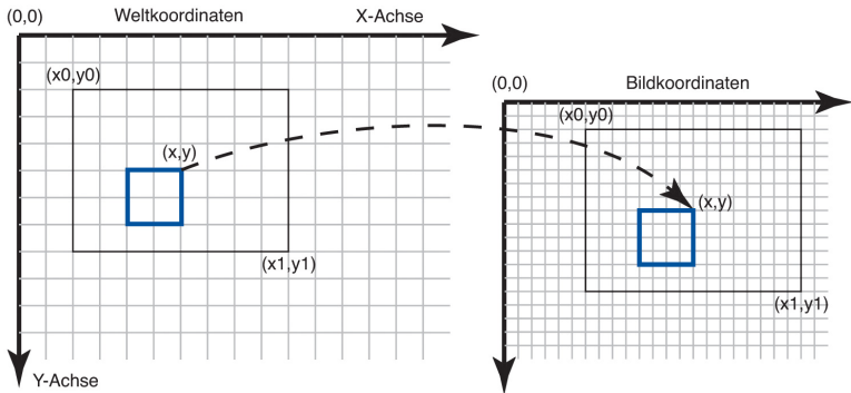
Abbildung 7.8: Transformation von Weltkoordinaten in Bildkoordinaten
