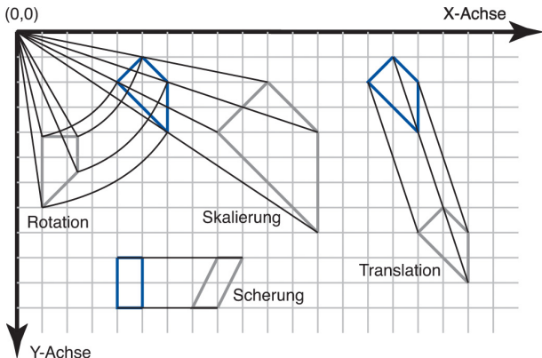
Abbildung 7.4: Die elementaren linearen Transformationen
