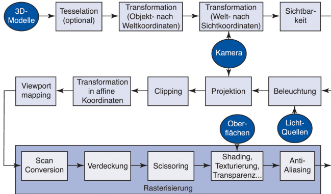
Abbildung 8.5: Die 3D Rendering Pipeline: der Weg vom 3D-Modell zum Bild unter Verwendung der Kamera, Lichtquellen und Oberflächenbeschreibungen
