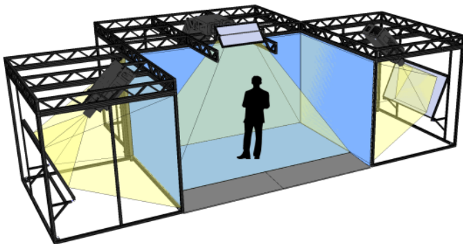
☞ Visbox: Schemazeichnung
