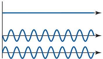
Destruktive Interferenz
