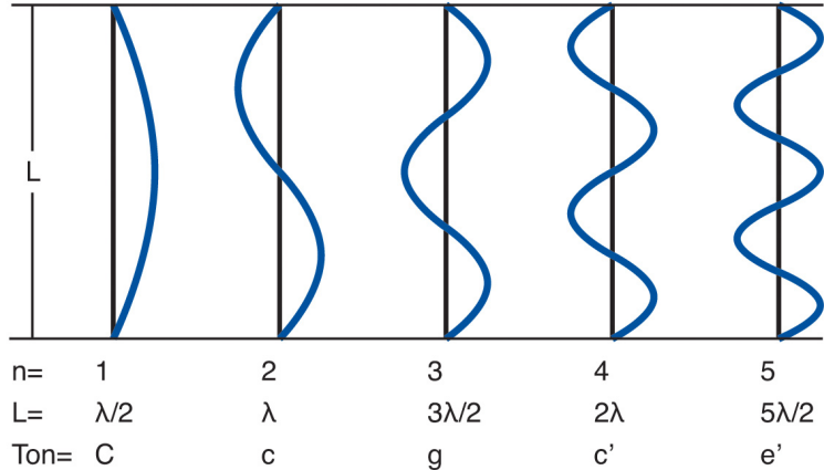
Abbildung 4.3: Oberwellen sind ganzzahlige Vielfache ( n ) einer Grundfrequenz.
