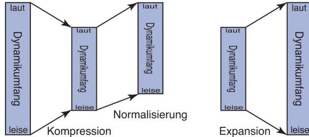
Abbildung 4.19: Kompression und Expansion der Dynamik eines Audiosignals
