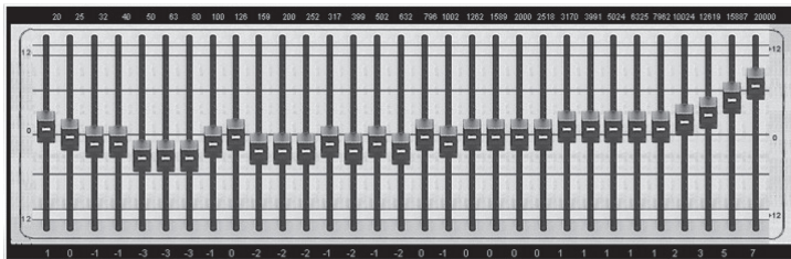
Abbildung 4.18: Grafischer Equalizer mit 31 Frequenzbändern im Abstand von jeweils einer Drittel Oktave
