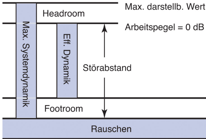
Abbildung 4.15: Headroom, Footroom, Dynamik und Störabstand eines Signals
