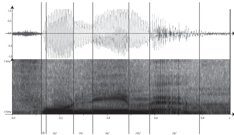
Abbildung 9.4: Wellenform und Frequenzspektrum des gesprochenen Wortes „Phoneme“. Dabei sind die einzelnen Phoneme des Wortes durch vertikale Linien abgegrenzt.
